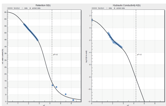
Abbildung 52: Wasserretentionskurve (links) und hydraulische Leitfähigkeit (rechts) für den A_{h,p} -Horizont von Bodenprofil 12 (Tiefe Zylinder 12–17 cm). Der pF -Wert ist der dekadische Logarithmus der Saugspannung in hPa. Messpunkte im gesättigten Bereich ( pF < 0.1 ) stammen vom KSAT-System, im feuchten Bereich ( pF 1–3.5) vom System HYPROP und im trockenen Bereich ( pF > 4 ) vom System WP4C.
