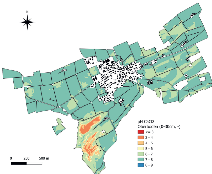
Abbildung 61: Regionalisierte Karte der pH-(CaCl 2 ) Werte für die Tiefenstufe 0–30 cm.
