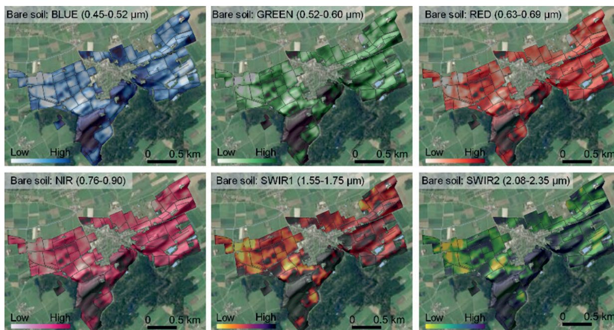
Abbildung 13: Bodenkartierung in Lommis: Spektrale Bodenlandschaftsanalyse des unbedeckten Bodens am Beispiel über 37 Jahre gemittelter Landsat-Spektralkanäle «BLUE», «GREEN», «RED», «NIR», «SWIR1» und «SWIR2».
