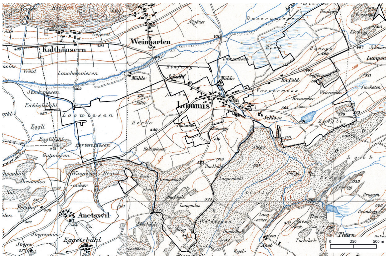
Abbildung 8: Auszug aus dem Topographischen Atlas der Schweiz (Siegfriedkarte) (Bundesamt für Landestopografie swisstopo), Erstausgabe von 1880. Der Projektperimeter ist in schwarz dargestellt.
