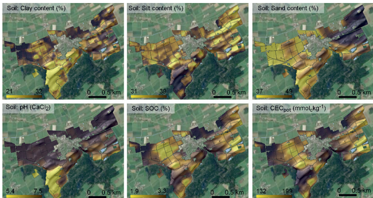
Abbildung 14: Indikative Bodeneigenschaftskarten am Beispiel der Tiefenstufe 0–30 cm und den Bodeneigenschaften Tongehalt («Clay content»), Schluffgehalt («Silt content»), Sandgehalt («Sand content»), pH-Wert («pH»), organischer Kohlenstoffgehalt («SOC») und potenzielle Kationenaustauschkapazität («CECpot»).
