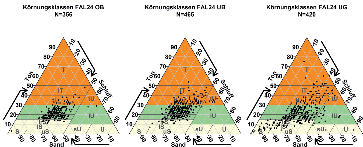
Abbildung 47: Körnungsdiagramme der Horizontdaten für die drei Bodenbereiche OB = Oberboden, UB = Unterboden, UG = Untergrund (N: Anzahl der Horizonte im jeweiligen Bodenbereich).
