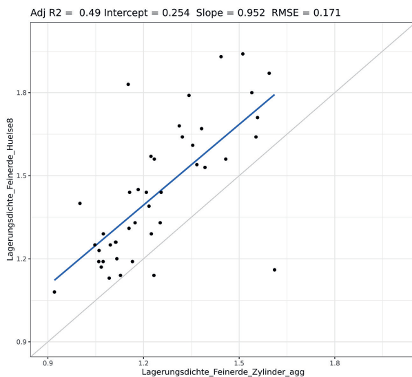
Abbildung 55: Vergleich der Lagerungsdichte Feinerde bestimmt mit 8 cm Hülsen und 100 ml Zylinderproben (links); Korrigierte Lagerungsdichte der 8 cm Hülsenproben und Lagerungsdichte bestimmt mit 100 ml Zylinderproben (Korrekturfaktor: 1.165).
