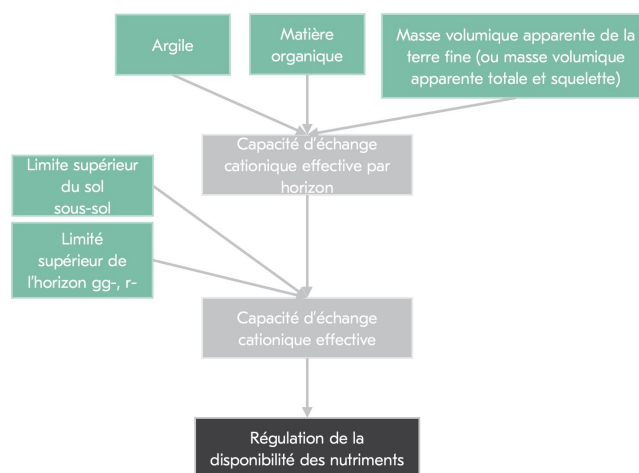
Figure 3 : Elaboration de la carte thématique pour la régulation de la disponibilité des nutriments.
