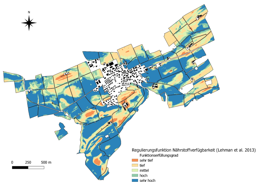
Figure 4 : Application de la méthode d'évaluation de la fonction de régulation pour la disponibilité des nutriments de la zone pilote de Lommis (TG).
