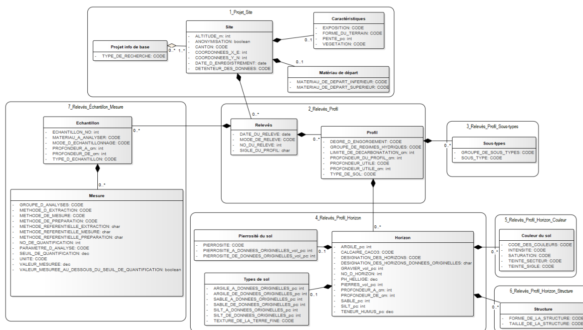
Figure 3 : Subdivision du fichier de données en 7 tableaux. Les liens entre les tableaux indiquent les relations qui existent entre les tableaux.
