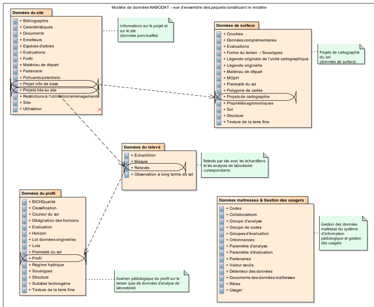
Figure 1 : NABODAT modèle de données valable à partir de la version 1.8 au niveau hiérarchique supérieur : vue d'ensemble des paquets et des liens.
