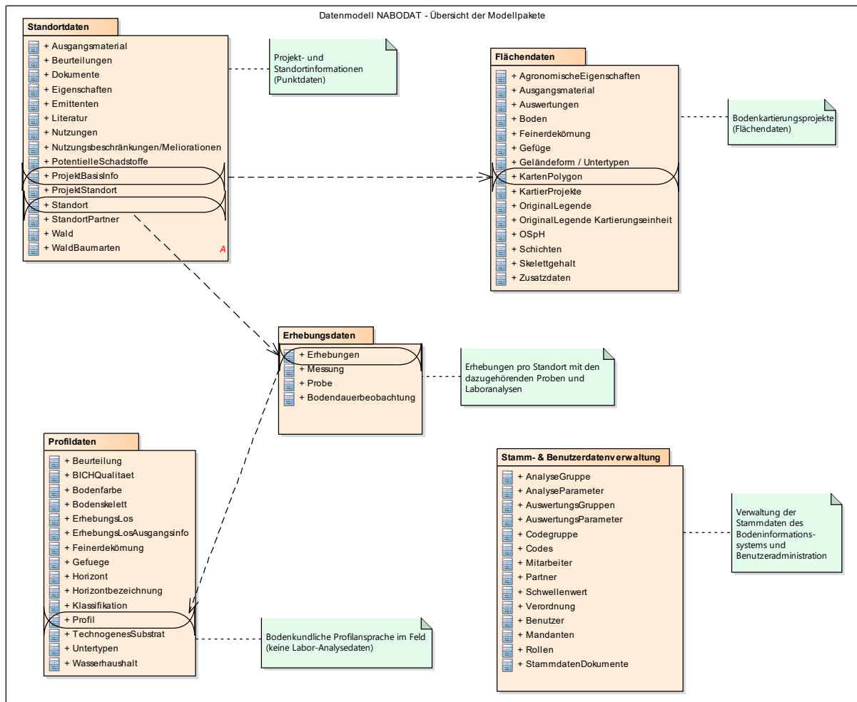
Abbildung 1: NABODAT Datenmodell gültig ab Version 1.8 auf der höchsten hierarchischen Stufe: Übersicht zu den Paketen und Verknüpfungen.
